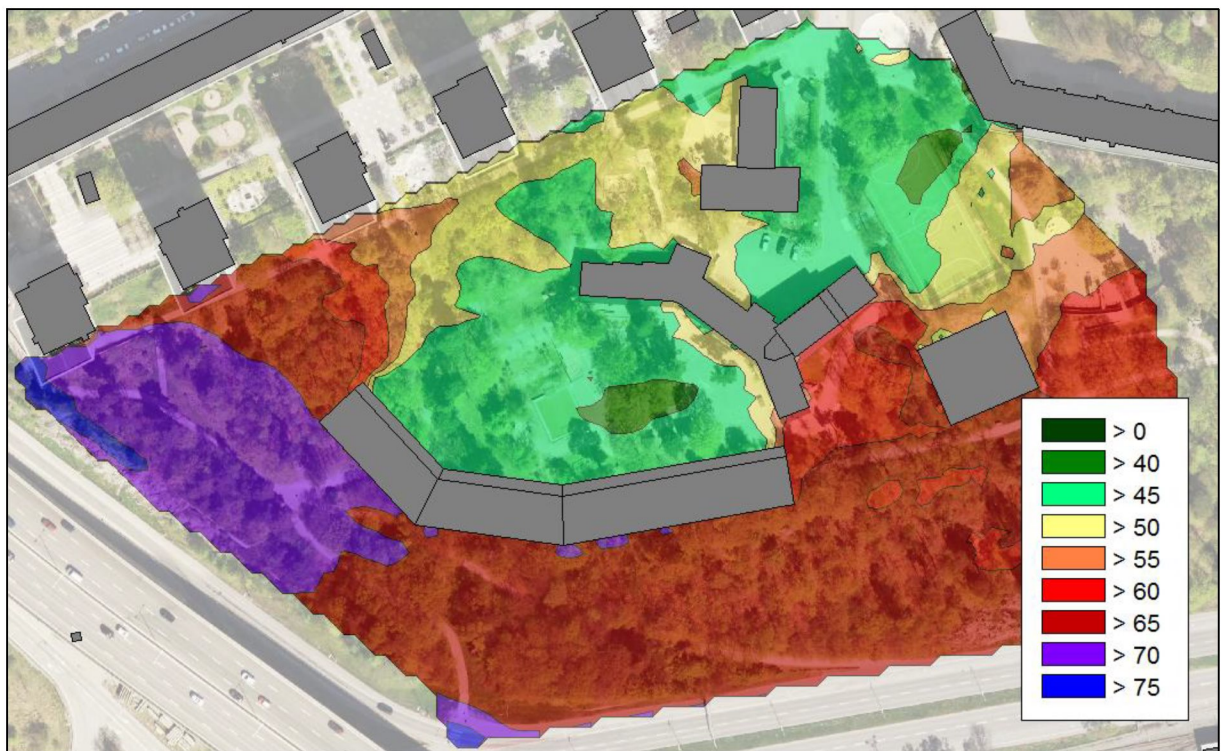
Figur 5 – Förslag I - Ekvivalenta trafikbullernivåer prognosår 2030 (dBA, L_{eq,24h} ).
