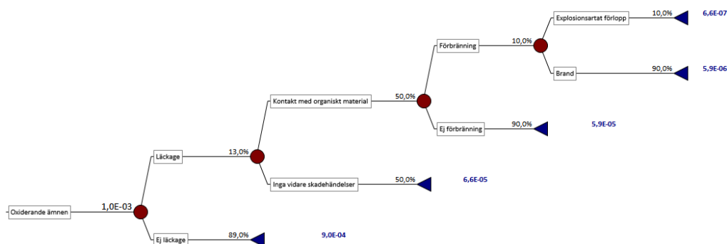
Figur A6. Händelseträd för oxiderande ämnen. Frekvenser för olika händelser redovisas i slutet av händelseträdets (per år). Notera att frekvenser som redovisas i händelseträdets baseras på 2 promille fordon lastade med farligt gods på sträckan.
