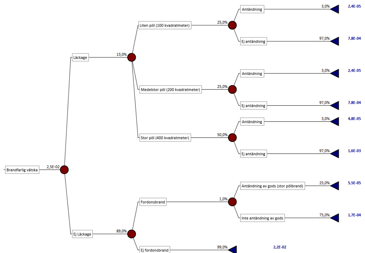
Figur A5. Händelseträd för brandfarlig vätska. Frekvenser för olika händelser redovisas i slutet av händelseträdets (per år). Notera att frekvenser som redovisas i händelseträdets baseras på 2 promille fordon lastade med farligt gods på sträckan.
