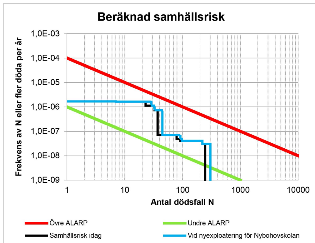
Figur 9. Beräknad samhällsrisk för dagens läge samt planerad utökning av detaljplaneområdet.
