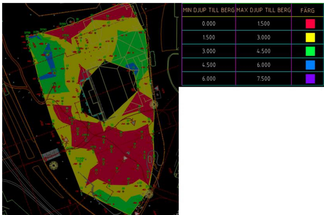
Figur 5. Djup till tolkad och interpolerad bergöverty från inmätt markyta i samband med inmätning av utförda borrpunkter.
