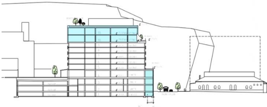
Figur 5. Typsektion befintlig konstruktion och planerad utbyggnad av Globen Shopping.
