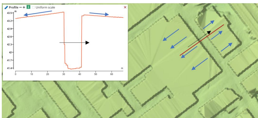
Figur 13 Höjdmmodell för befintligt scenario över Kv. A och befintligt hus för läget av Dp2d, blå pilar visar flödesriktning och svart pil hur den röda profilen är dragen. Utdrag från Scalgo.
