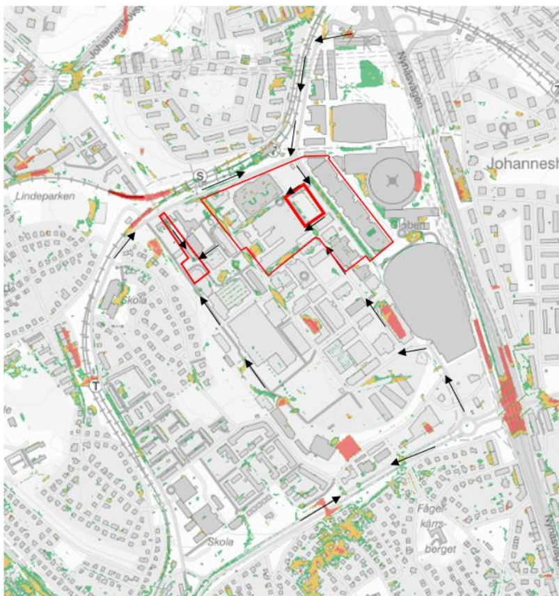
Figur 37 Svarta pilar redovisar möjliga tillfartsvägar för räddningstjänstfordon till Dp2a, Dp2c, Dp2d samt Slakthusområdet i stort. Gröna ytor redovisar översvämmande ytor vid skyfall med ett vattendjup på 0,1-0,2 m, gula på 0,2-0,5 m och röda över 0,5 m vattendjup (röda ytor som är överstreckade är översvämmande underfarter)
