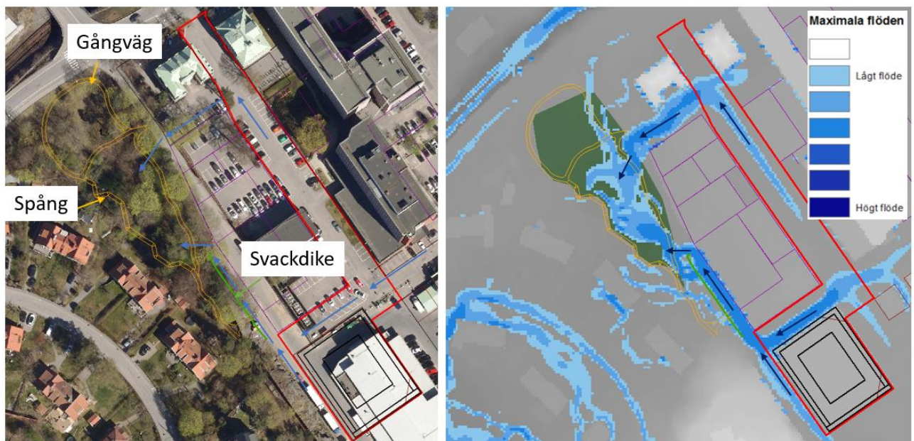
Figur 29 Till vänster visas åtgärder för att leda skyfallsvattnet till lågpunkten i Frötallen, grön linje markerar läget för svackdiket, orangea linjer markerar upphöjd gångväg samt spång och blå pilar markerar flödesriktning. Till höger beräknade flöden med åtgärderna inkluderade.
