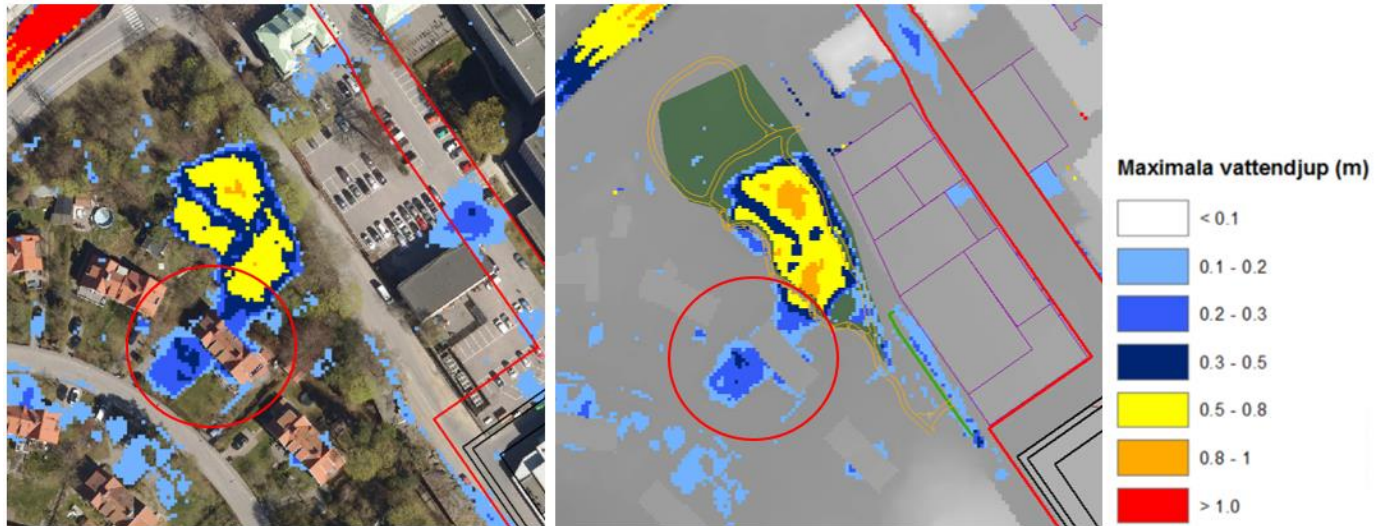
Figur 30 Översvämningsutbredning inom Frötallen och vid byggnad längs Livdjursgatan, vill vänster vid befintligt scenario och till höger med ny exploatering, röd cirkel markerar byggnad som riskerar att drabbas av översvämning vid skyfall.
