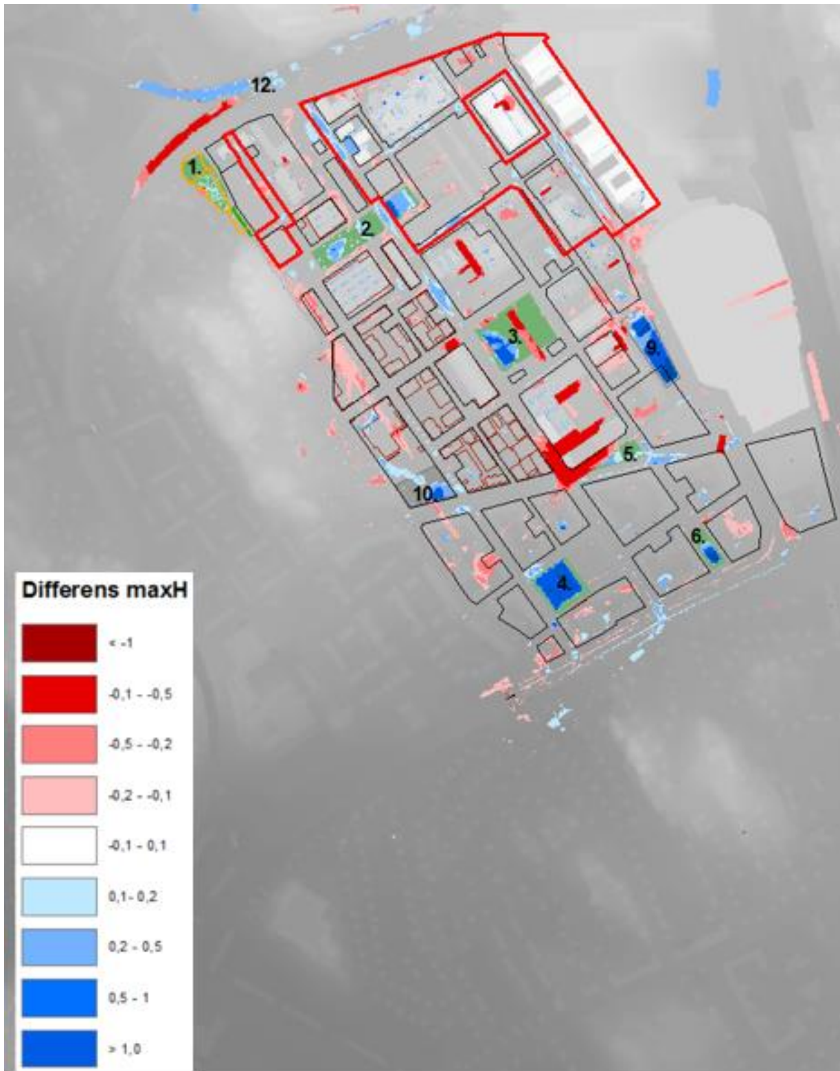
Figur 36 Differenskartan, redovisar skillnader i beräknade vattendjup mellan befintligt scenario och med ny exploatering. Rött visar att det är mer vatten i befintligt scenario blått visar att det är mer vatten vid ny exploatering. Röda linjer visar detaljplanegränserna för Dp2a, Dp2c och Dp2d. Observera att det är vattendjup och inte vattennivå.
