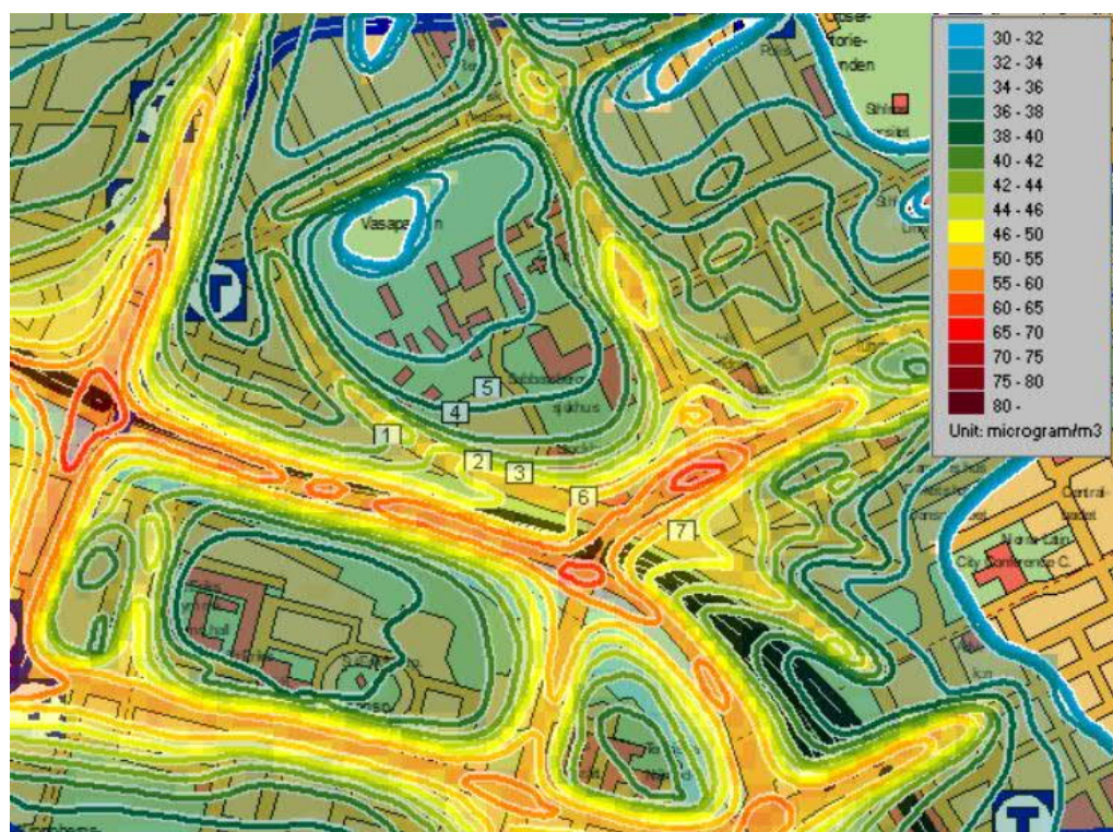
Figur 16 Beräknade halter av NO 2 som timvärden (98h) år 2030. Halter enligt färgskalan [µg/m 3 ]. MKN = 90 [µg/m 3 ] och MKM = 60 [µg/m 3 ].
