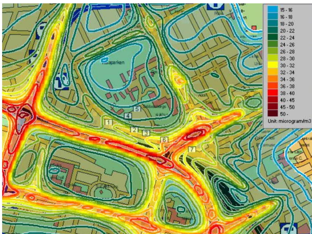
Figur 15 Beräknade halter av NO 2 som dygnsvärden (98D) år 2030. Halter enligt färgskalan [µg/m 3 ]. MKN = 60 [µg/m 3 ].
