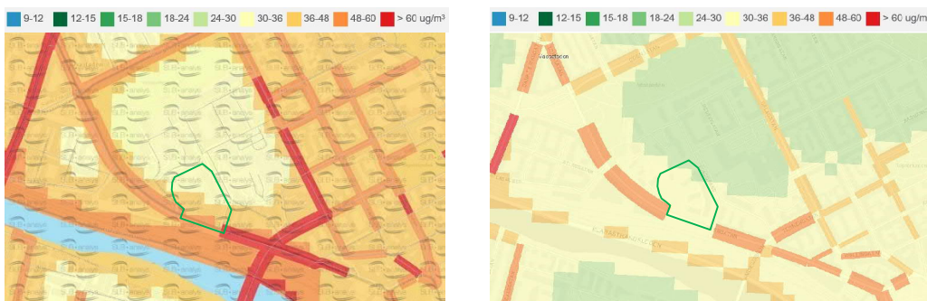
Figur 4 Översiktliga beräkningar av NO 2 dygnsvärden för år 2015 (vänster) och 2020 (höger). Utdrag ur publicerade föroreningskartor (ÖSLVF, 2021). Grön figur visar planområdet.
