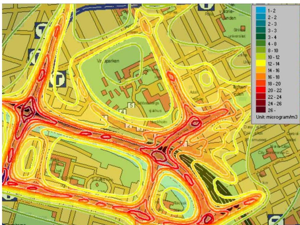
Figur 14 Beräknade halter av NO 2 år 2030 som årsmedelvärde. Halter enligt färgskalan [ \mu\text{g}/\text{m}^3 ]. MKN = 40 [ \mu\text{g}/\text{m}^3 ] och MKM = 20 [ \mu\text{g}/\text{m}^3 ].
