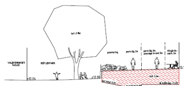
Sektion B-B
