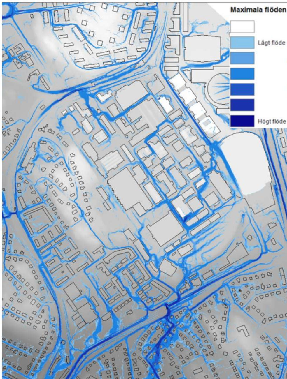
Figur 7 Nulägesmodellering, beräknade maximala flöden (m 3 /s/m) under hela simuleringen vid ett klimatkorrigerat 100-årsregn. (Uppdaterad 2022-04-01).
