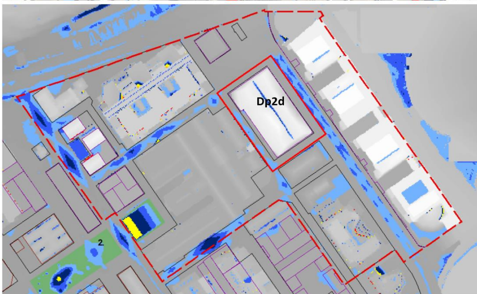
Maximala vattendjup (m)
