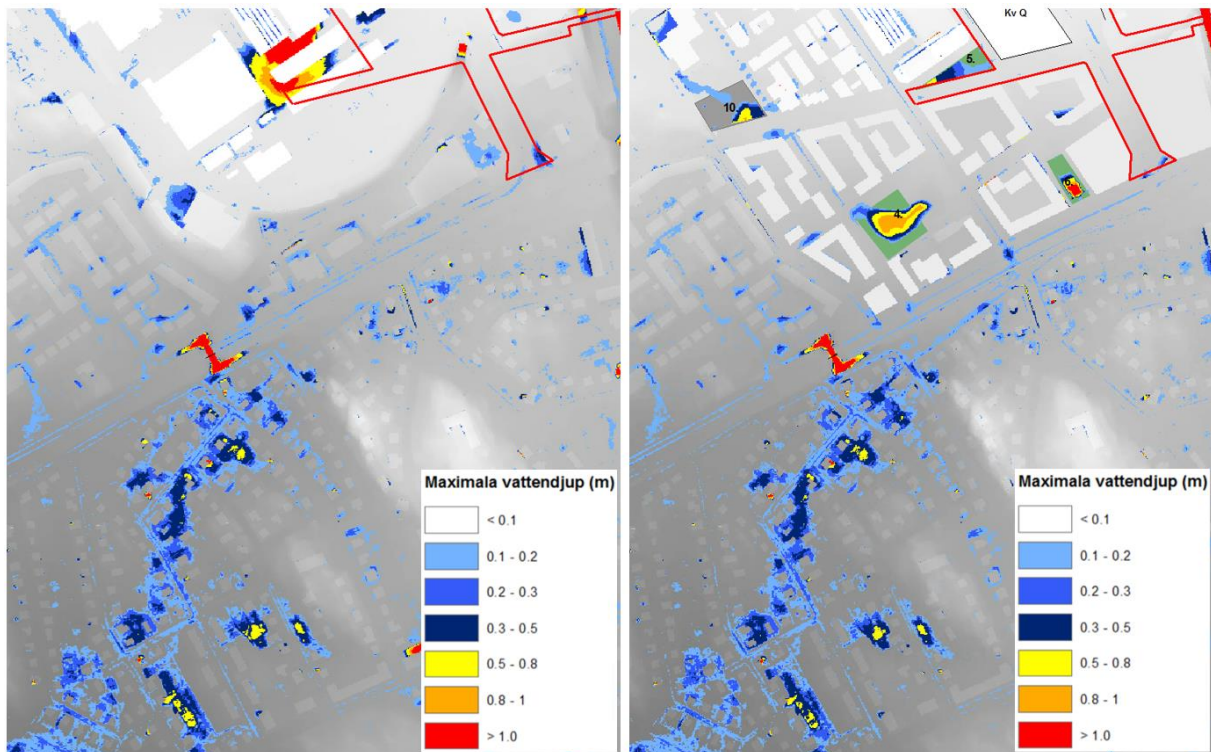
Figur 39 Beräknade maximala vattendjup i, till vänster vid befintligt scenario och till höger vid ny exploatering. (Uppdaterad 2022-04-01)
