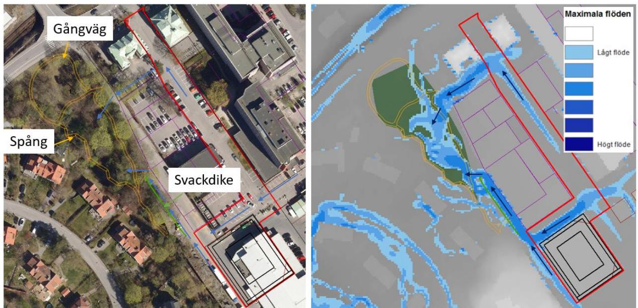
Figur 35 Till vänster visas åtgärder för att leda skyfallsvatten till lågpunkten i Frötallen, grön linje markerar läget för svackdiket, orangea linjer markerar upphöjd gångväg samt spång och blå pilar markerar flödesriktning. Till höger beräknade flöden med åtgärderna inkluderade.
