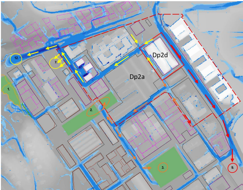
Figur 33 Hantering av skyfallsvatten från Dp2a. Skyfallsvattnet hanteras i nr 2: Östra och Västra Fållan (utreds i detaljprojektering om mer vatten kan ledas dit inom Dp2), se orangea pilar samt i nr: 3 Centrala parken, nr:7, Slakthusplan se gula pilar (utreds hur mycket som kan tas omhand där inom Dp5), det vatten som inte ryms inom Slakthusplan och i östra respektive västra Fållan leds till befintligt spårområde och under överdäckningen inom Dp5b, nr: 12. och vattnet som rinner söderut längs Arenavägen och Rökerigatan röda pilar, hanteras på Evenemangstorget inom Dp4.
