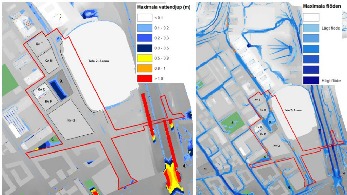
Figur 31 Till vänster beräknade maximala vattendjup inom Dp4a och till höger flödesvägar till och inom Dp4a. Den röda vattenansamlingen till höger visar att det samlas vatten i lågpunkten på Nynäsvägen, ingår ej i Dp4a)
