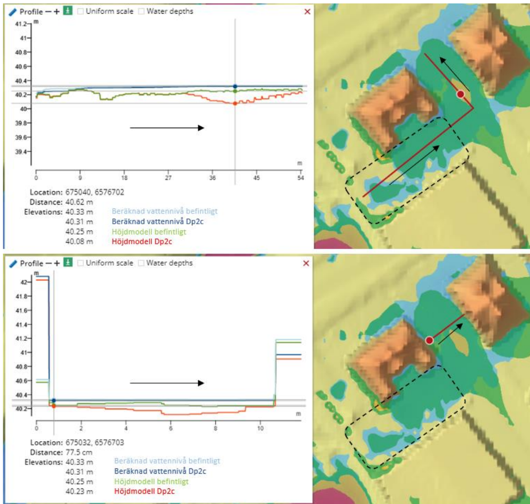
Figur 20 Beräknad vattennivå vid Kylhuset 15. I den övre bilden redovisas beräknade vattennivåer i en profil i gatans mitt och i den nedre bilden i en profil för en tvärsektion över gatan. Blå yta är översvämningsutbredning vid befintligt scenario och grön/gul/röd är med vid ny exploatering (endast vattendjup över 5 cm redovisas). Svarta pilar visar i vilken riktning profilen är dragen. Inom den streckade ytan har befintlig höjsättning använts (området är en del av Dp5a).
