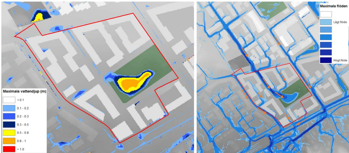
Figur 28 Till vänster beräknade vattennivåer inom Dp3 och till höger flödesvägar till och inom Dp3 vid ny exploatering enligt Dp3
