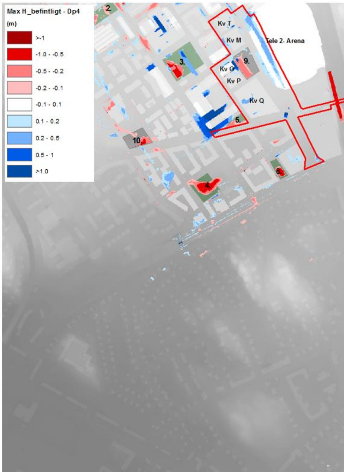
Figur 40 Differenskartan, redovisar skillnader i beräknade vattendjup mellan befintligt scenario och med ny exploatering. Blått visar att det är mer vatten i befintligt scenario rött visar att det är mer vatten vid ny exploatering. Röda linjer visar detaljplanegränserna för Dp4a.
