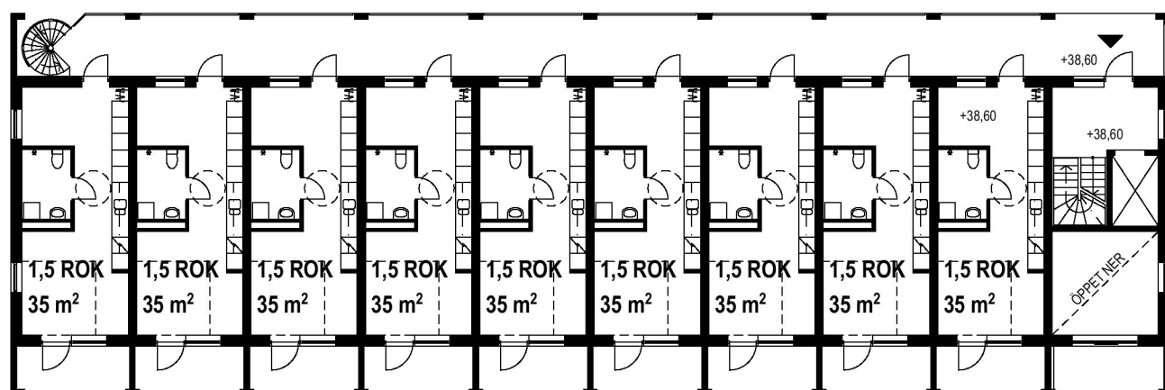
Entréplan, Hus F Skala 1:250 (A3)
