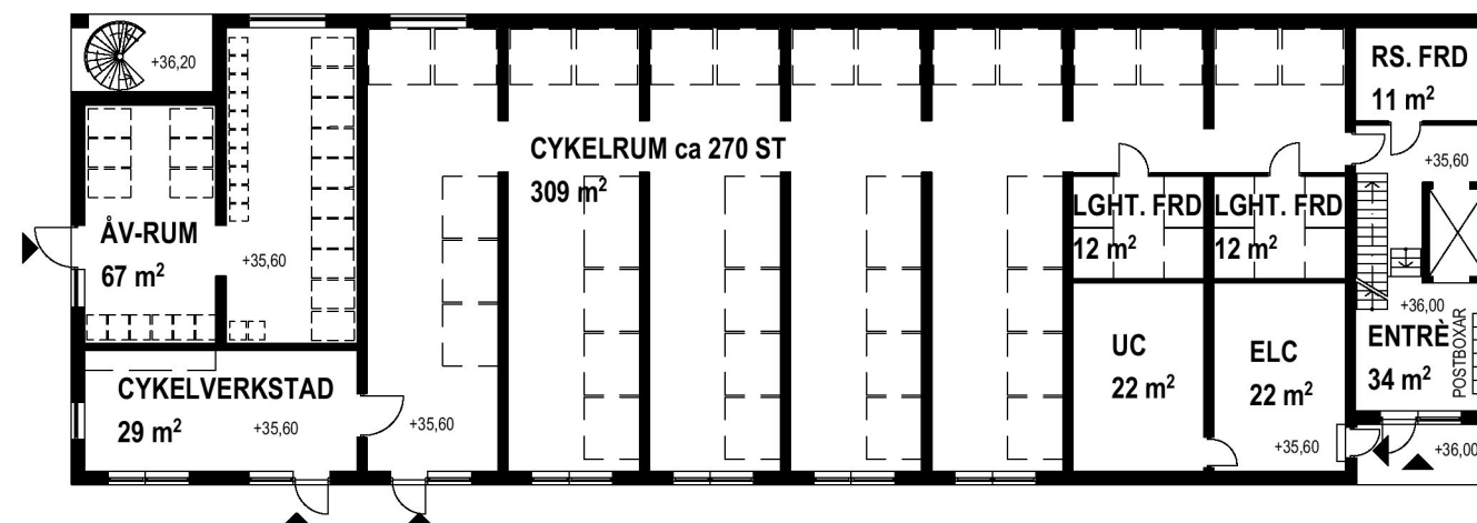
Källarplan, Hus F Skala 1:250 (A3)
