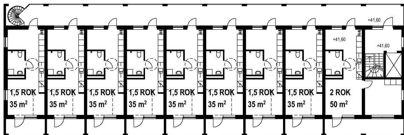
Normalplan, Hus F Skala 1:250 (A3)
