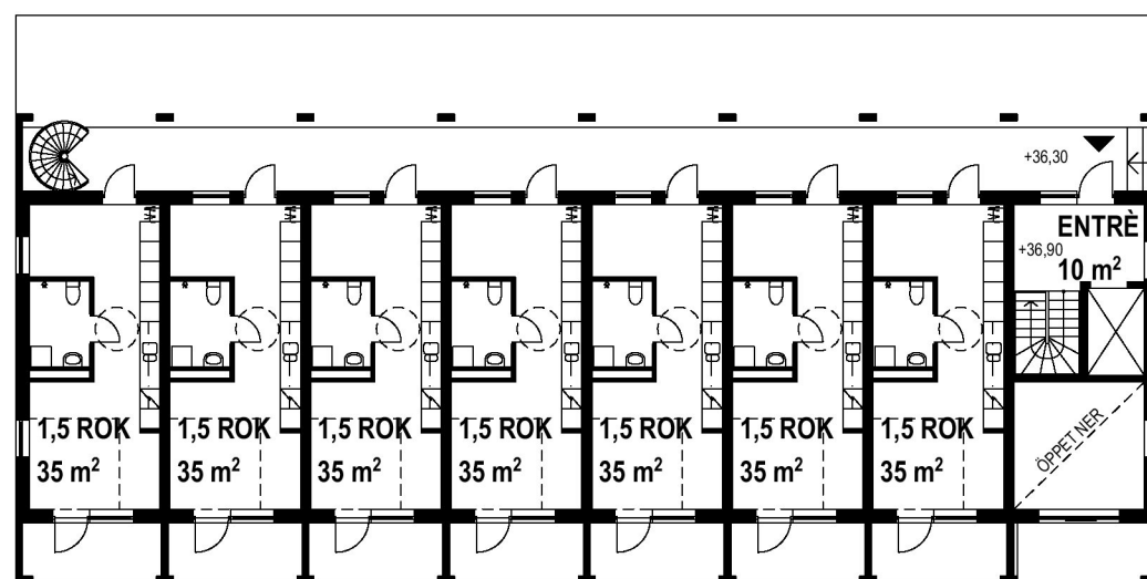
Entréplan, Hus E
