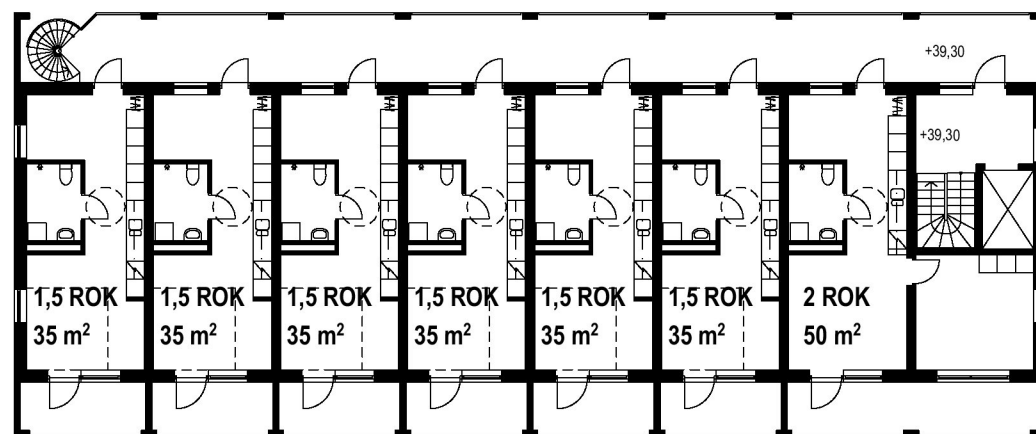
Normalplan, Hus E
