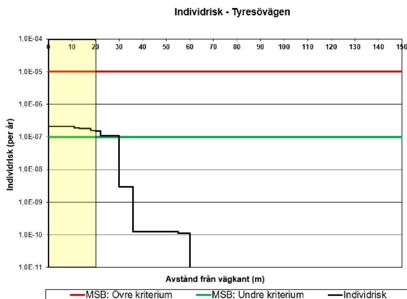
Figur 5.2. Individrisk prognos år 2040 utmed Tyresövägen. Markering visar kortaste avstånd till bebyggelse (parkeringshuset). (Observera att frekvensen redovisas med logaritmisk skala.)
