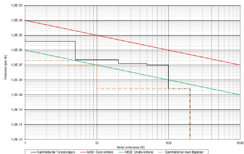
Figur 5.1. F/N-kurva som redovisar samhällsrisknivån då transporter med gasol i flaskor byts mot fordonsgastransporter i tankbil. Samhällsrisknivån beaktat de säkerhetshöjande åtgärderna som föreslås redovisas också utifrån den förändringen.
