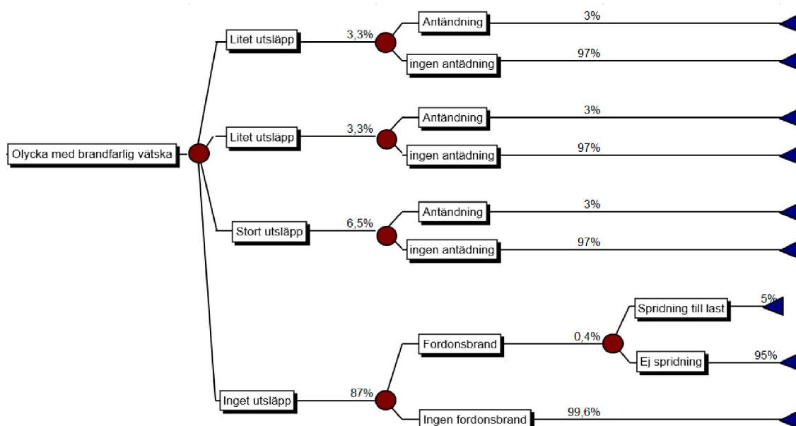
Figur A.2. Händelseträd olycka med transport av brandfarlig vätska (klass 3).
