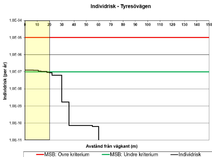
Figur 5.1. Individrisk i nuläge utmed Tyresövägen. Markering visar kortaste avstånd till planerad bebyggelse (parkeringshus). (Observera att frekvensen redovisas med logaritmisk skala.)
