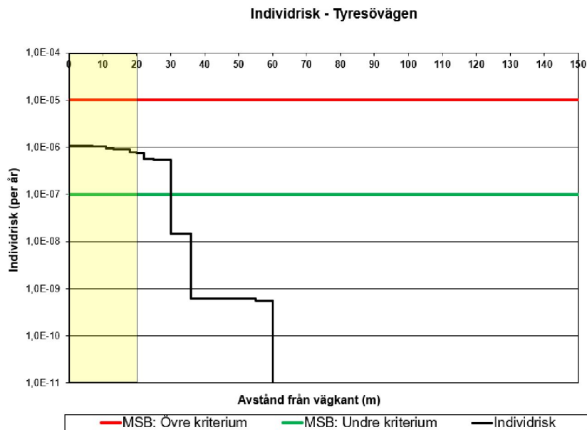
Figur 5.1. Individrisk utmed Tyresövägen beaktat att transporter av farligt gods femfaldigas.
