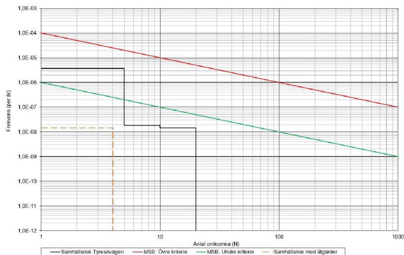
Figur 5.1. F/N-kurva som redovisar samhällsrisknivån enligt figur 5.3 tillsammans med F/N-kurva för samhällsrisk beaktat effekten av de åtgärder som föreslås.
