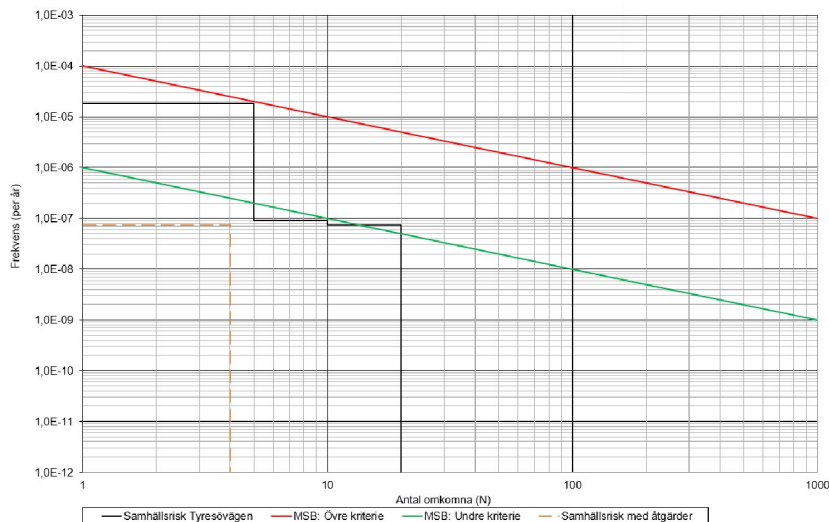
Figur 5.1. F/N-kurva som redovisar samhällsrisknivån om antalet transporter femfaldigas. Samhällsrisknivån beaktat de säkerhetshöjande åtgärderna som föreslås redovisas också utifrån den ökningen.
