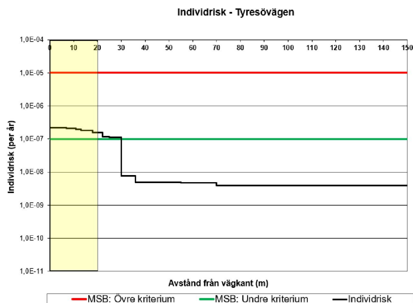
Figur 5.1. Individrisk utmed Tyresövägen då transporter med gasol i flaskor byts mot fordonsgastransporter i tankbil.
