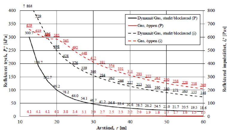
Figur 14 Resultande last från reflekterad luftstötavgång orsakad av 100 kg dynamit, starkt blockerad gasexplosion samt gasexplosion på öppen yta.
