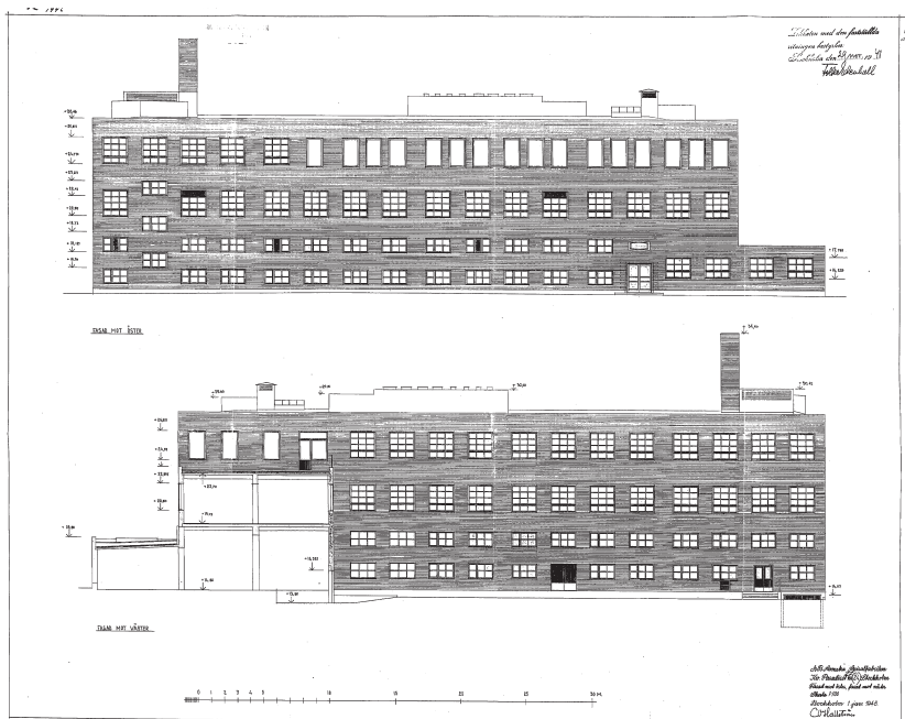
Ritning från 1948 som visar Svenska Spiralfabriken's huvudbyggnads östra och västra fasader. Källa: SBK.
