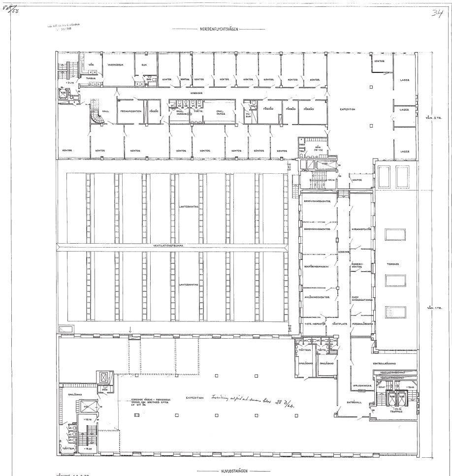
Jämförelse mellan ritningarna för Svenska Spiralfabrikens byggnad (övre) och Pressbyråns byggnad (nedre), båda visar våning 1 trappa. Observera den bevarade skorstenen, trapphuset och schaktöppningen i nedre vänstra hörnet samt pelareplaceringarna. Källa: SBK.
