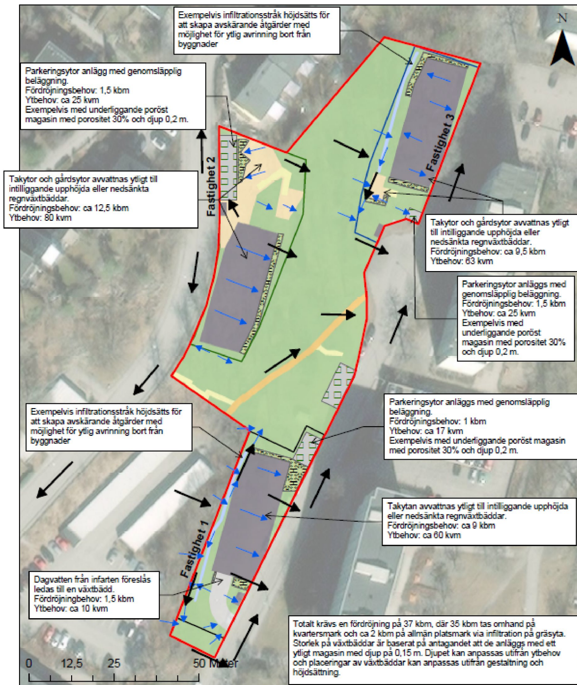
Illustration som visar förslag till hantering av dagvatten inom kvartersmarken. Illustration: Bjerking
