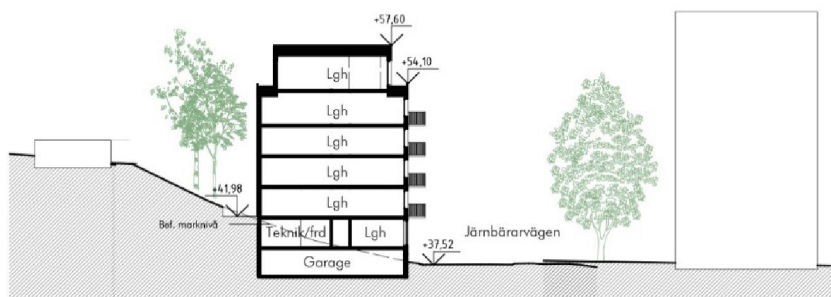
Sektion 1 A, genom Hus 1. AIX Arkitekter
