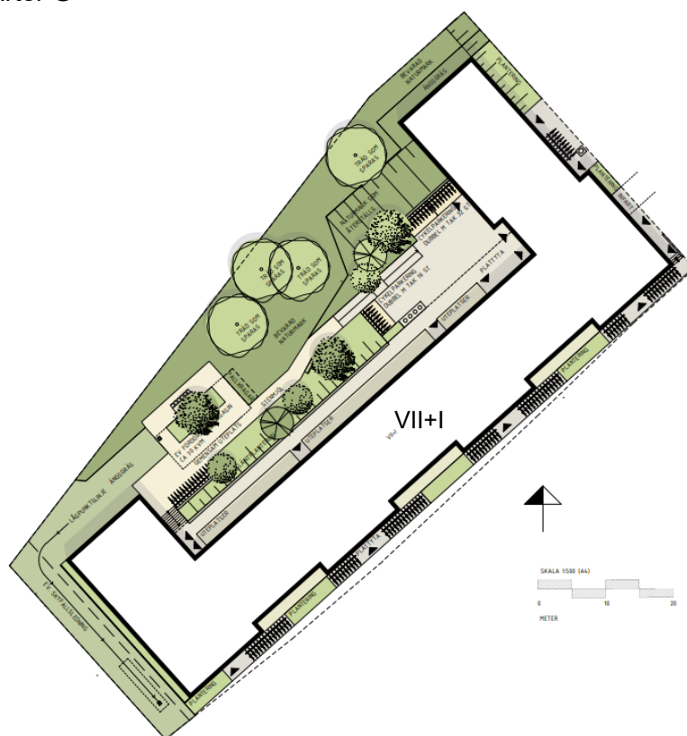
Situationsplan över kvarter G. Bild av Outerspace arkitekter.
