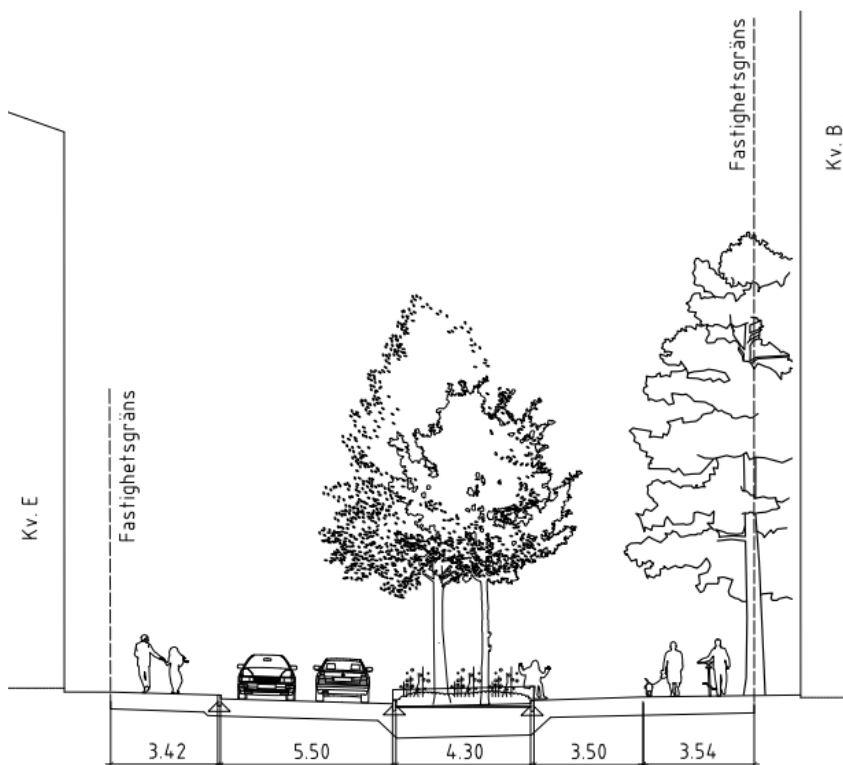
Gatusektion C, lokalgata från Skateparken mot Zeppelinargatan. Gatuavsnittet har en extra bred planteringszon. Bild av Nyréns.
