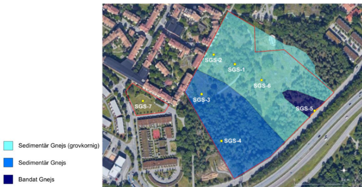
Berggrundkarta över planområdet. Bild av WSP.
