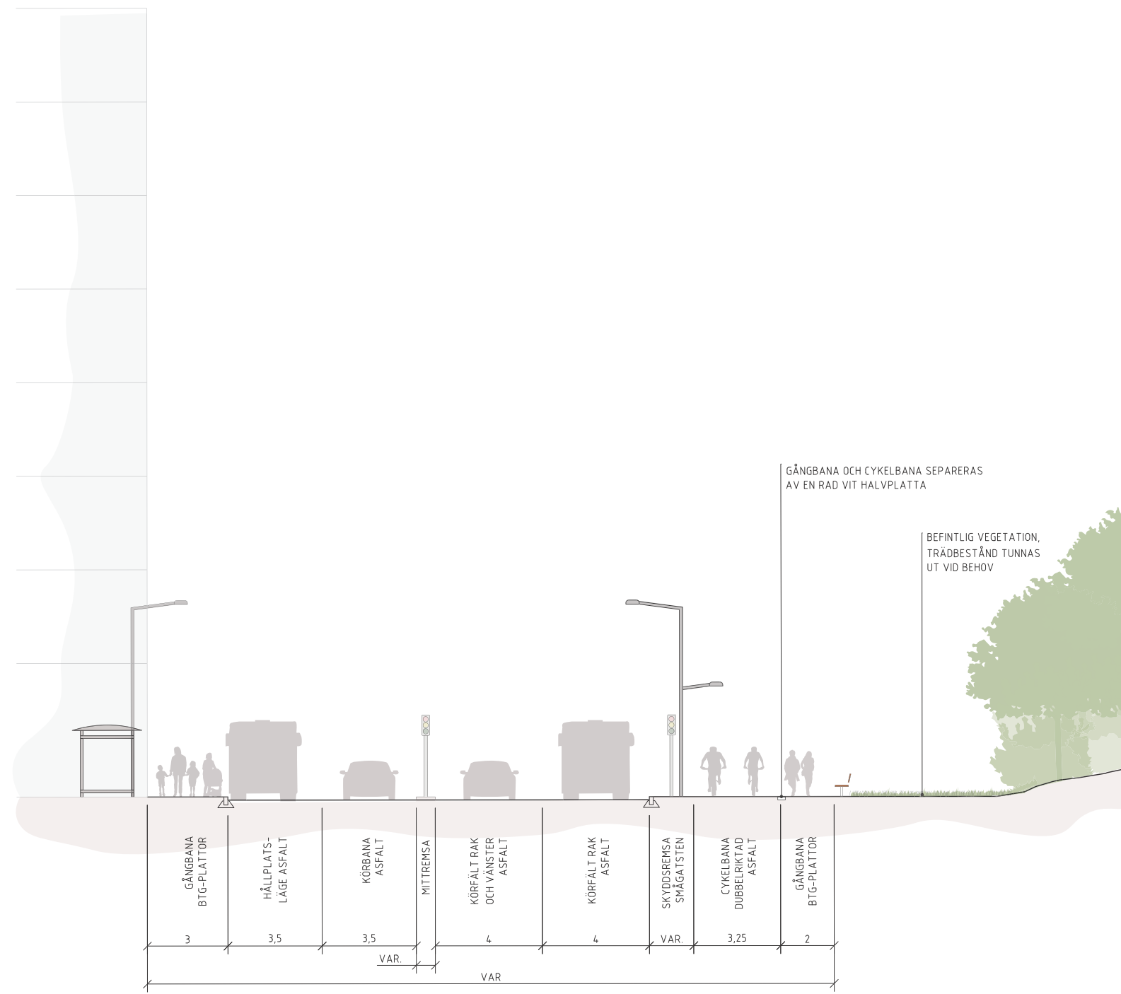
Magelungsvägen B-b
