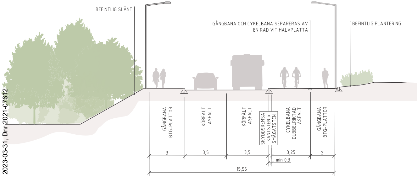
Magelungsvägen A-a
