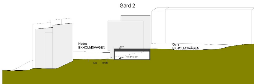
Sektion S4 genom gård 2
