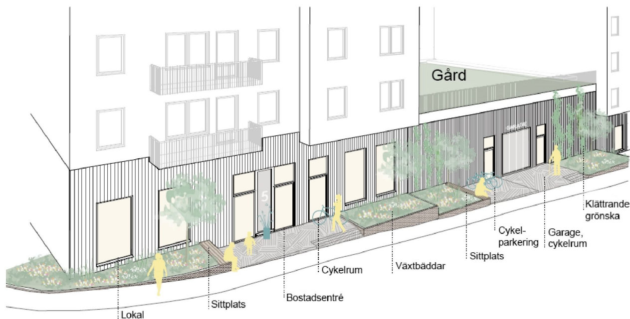
Utsnitt på sockenvåning mot nedre Ekholmsvägen.
