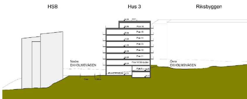
Sektion S5 genom hus 3
