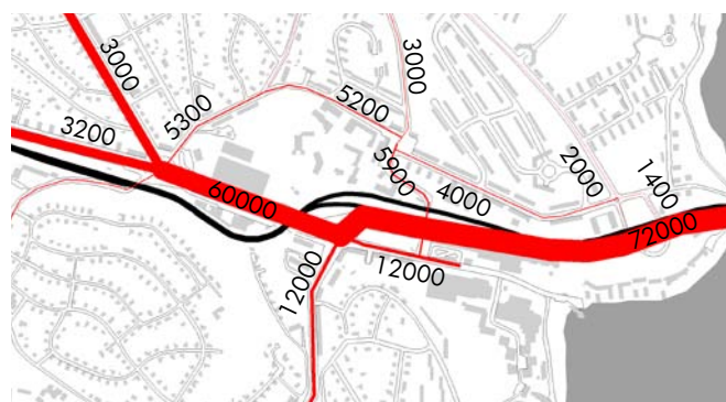
Trafikflödeskarta (antal bilar och bussar ett vardagsdygn under 2001-2002) Västerort - Trafikflödeskarta
