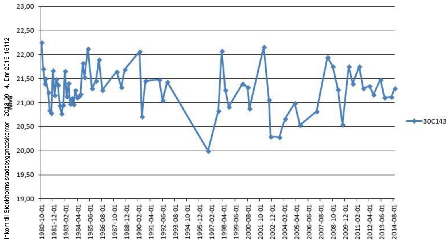
Grundvattenmätning för perioden från 1980-10-16 till 2014-09-30
