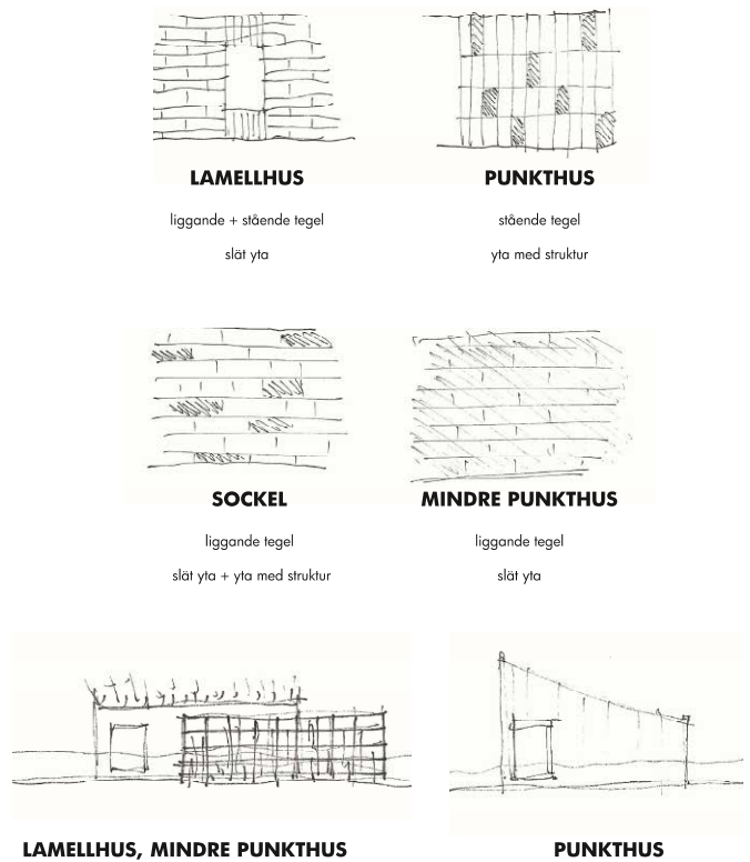
Princip tegelbearbetning och takvolym
