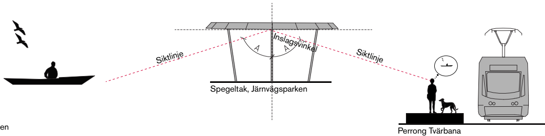
Bällstaviken Spegeltaket, så fungerar det.
