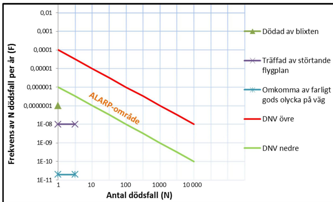
Figur 11: DNV:s FN-diagram rekommenderat av MSB, /Statens Räddningsverk 1997/.
