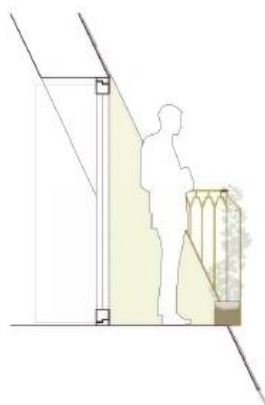
Sektionsutsnitt balkong i det vinklade taket. Bild: Marge
