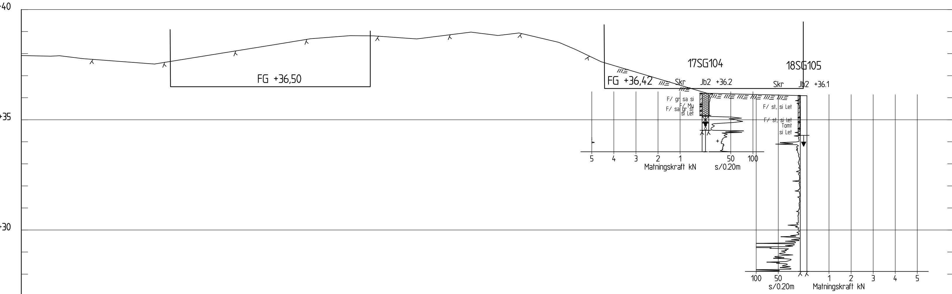
SEKTION C-C H 1: 100 L 1: 200
