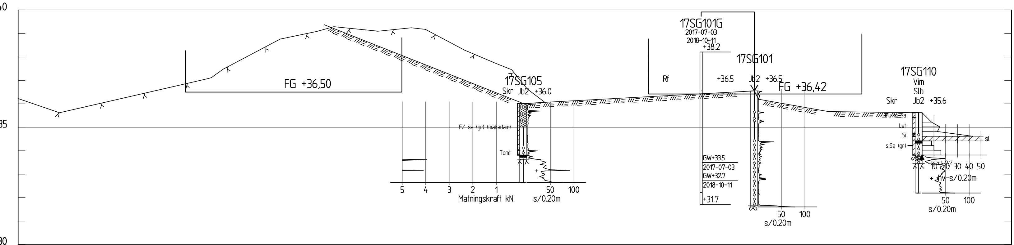
SEKTION C-C H 1: 100 L 1: 200
