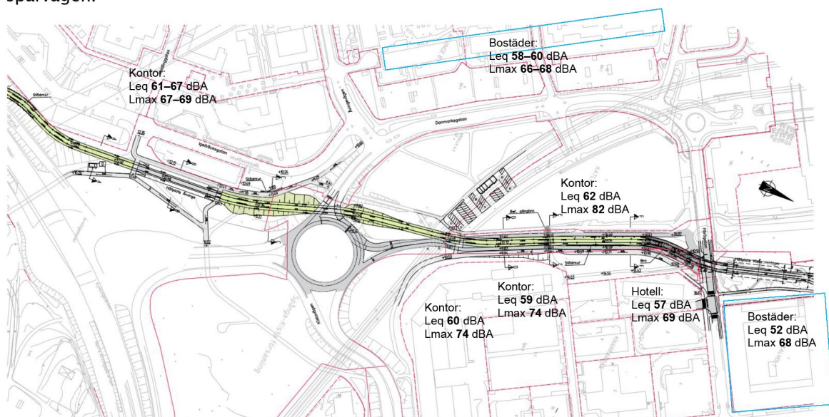
Figur 7. Beräknade ljudnivåer från vägtrafik (frifältsvärden vid fasad).
