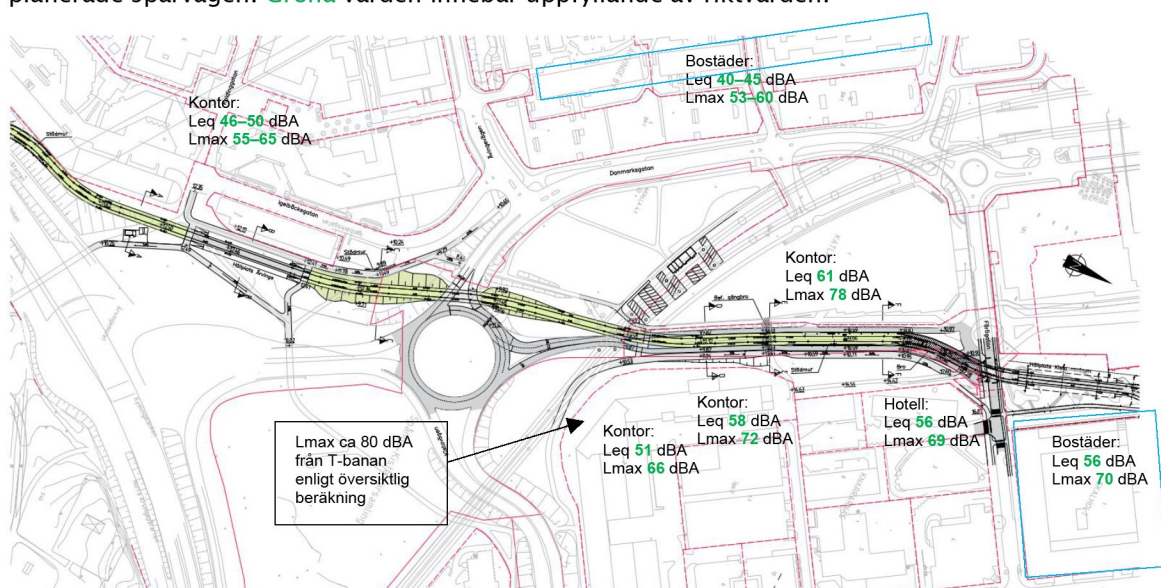
Figur 8. Beräknade ljudnivåer från Tvärbanan (frifältsvärden vid fasad).
