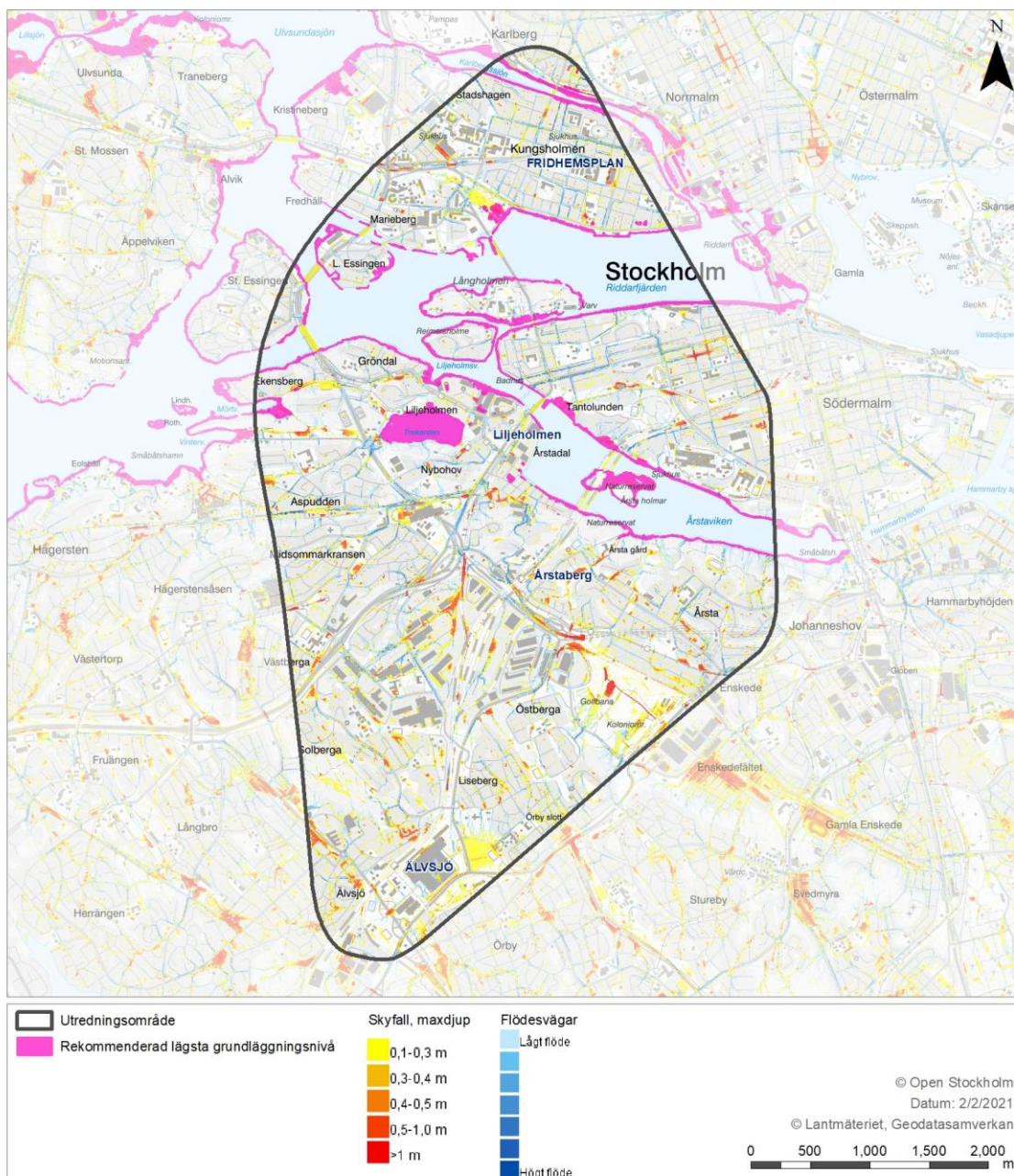
FIGUR 9. MAXIMALA VATTENDRUPOR OCH FLÖDEN VID ETT 100-ÅRSREGN (KÄLLA: STOCKHOLMS STADS SKYFALLSKARTERING) SAMT LÄNSSTYRELSENS REKOMMENDERADE LÄGSTA GRUNDLÄGGNINGSNIVÅ (+ 2,7 M I RH2000).
