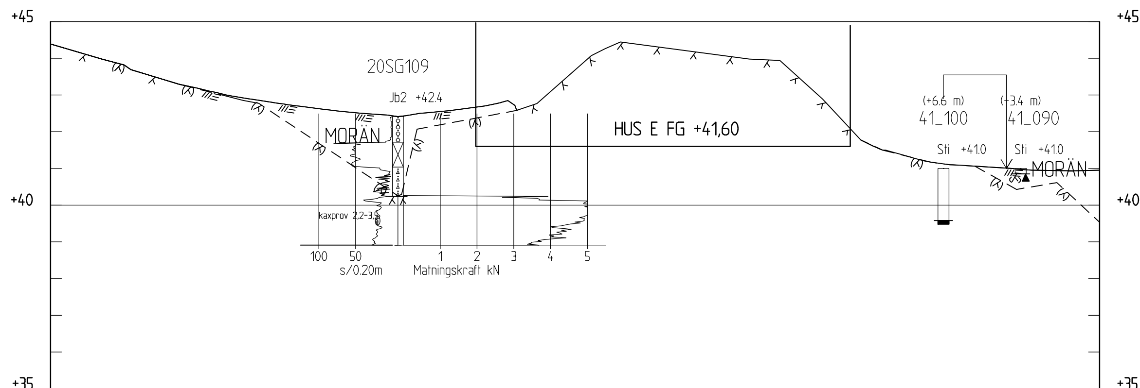
SEKTION H-H 1: 100
