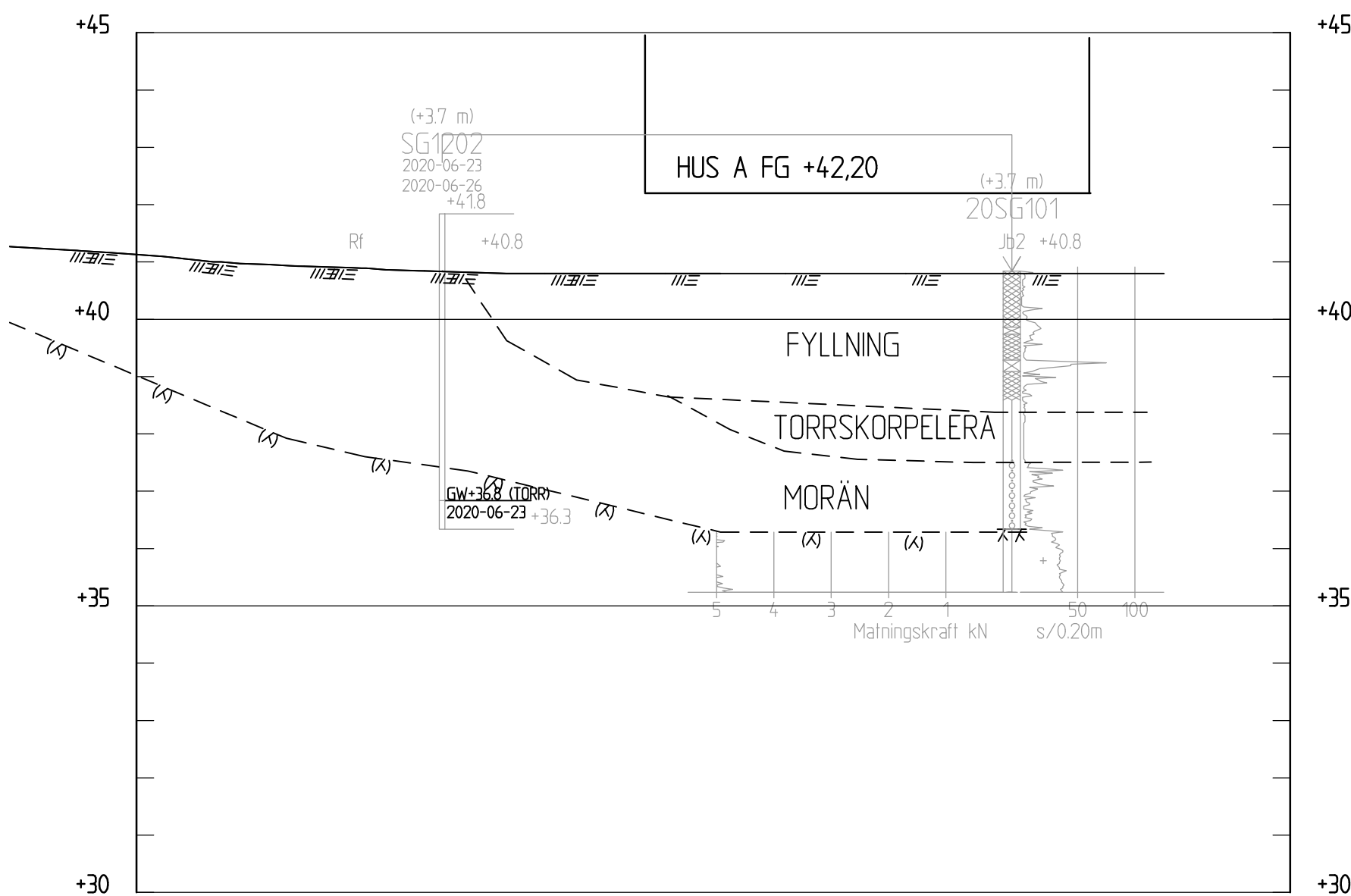
SEKTION E-E 1: 100
