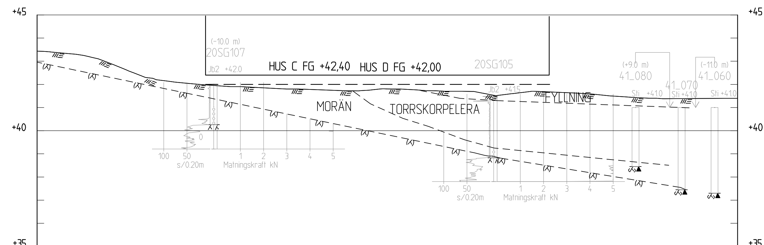
SEKTION I-1 1: 100
