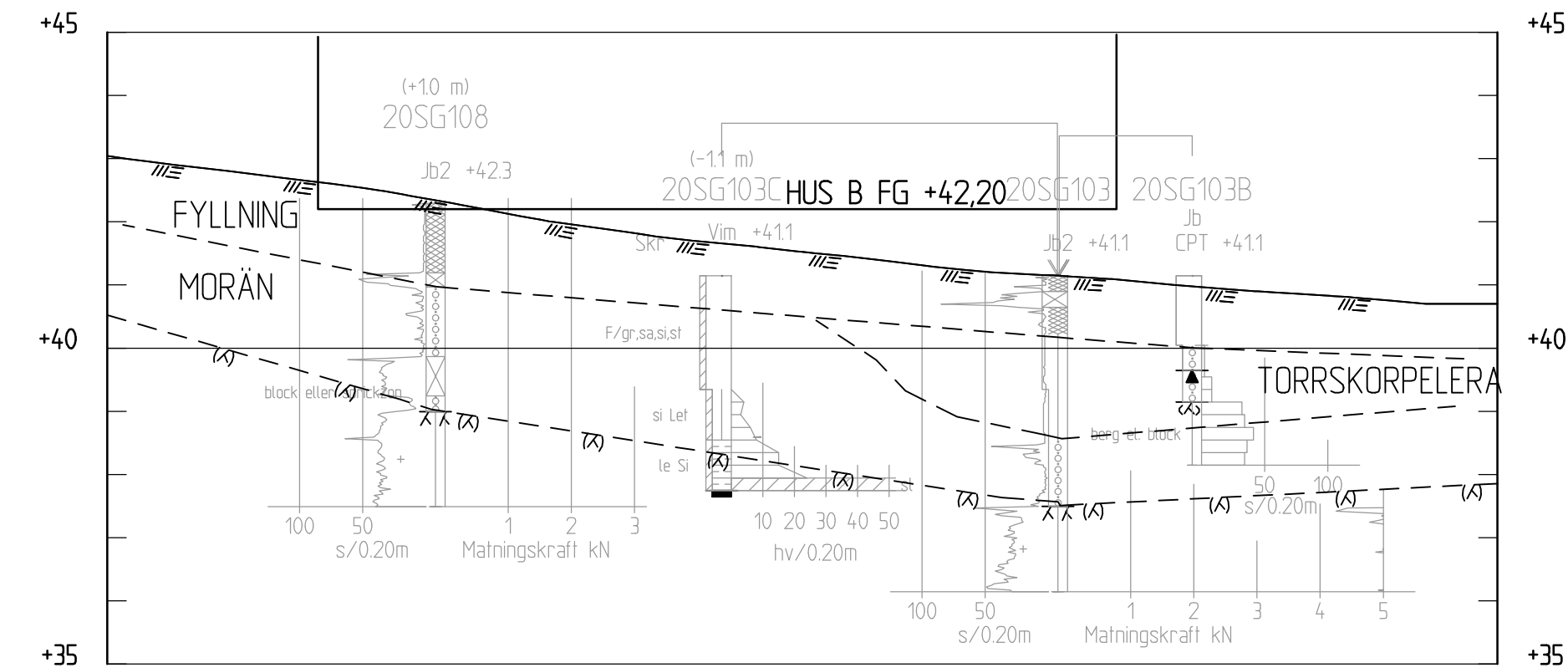
SEKTION C-C 1: 100
