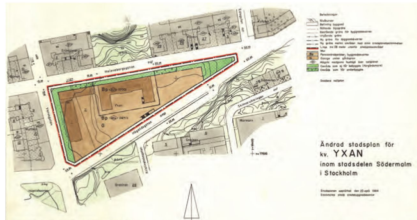
Plankarta 6285 (laga kraft 1964-07-10) för kv. Yxan inom stadsdelen Södermalm i Stockholm.
