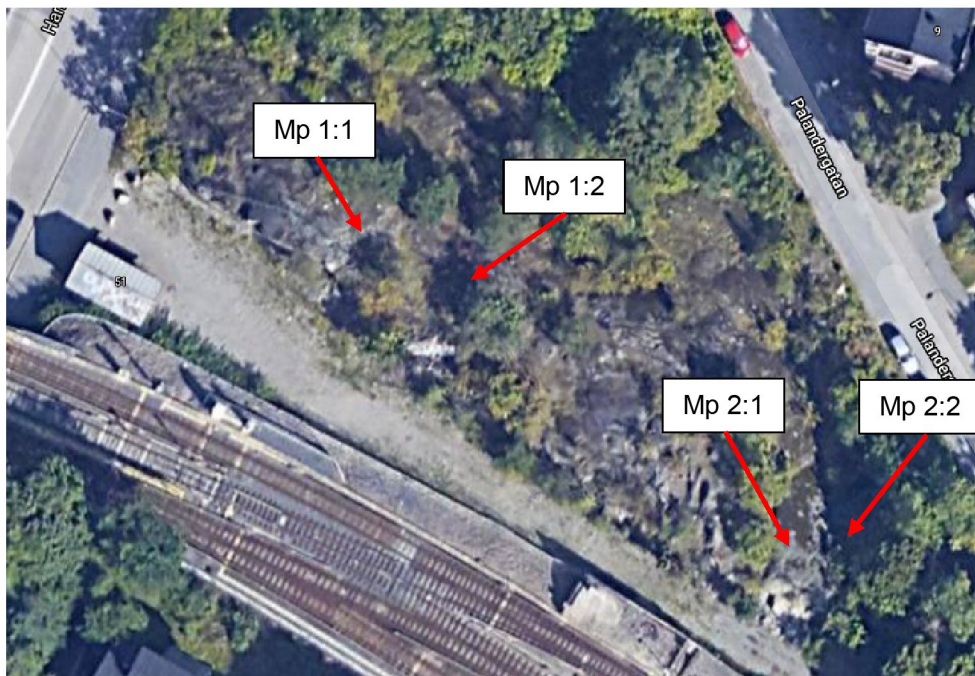
Figur 4 Mätpunkter
