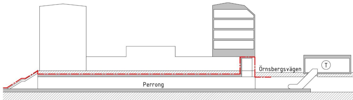
A-A
