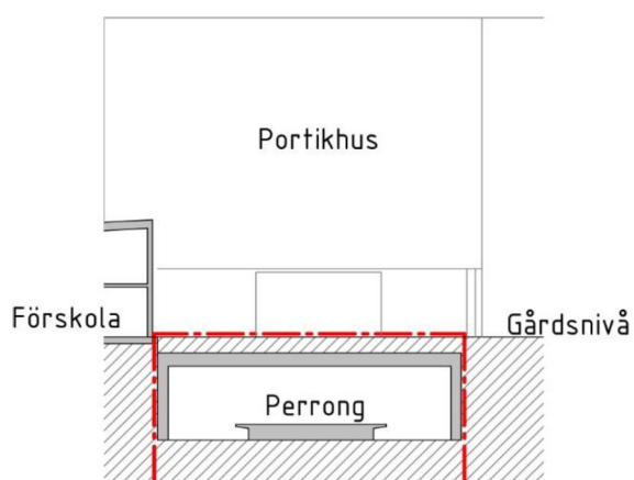
B-B
