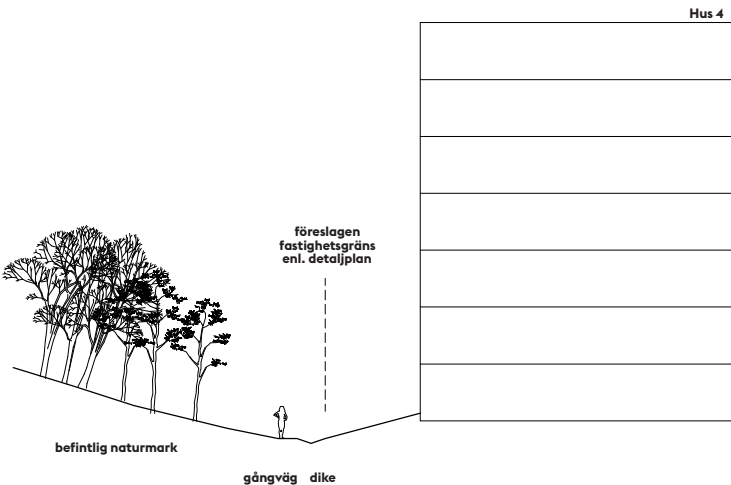
Sektion B-B
