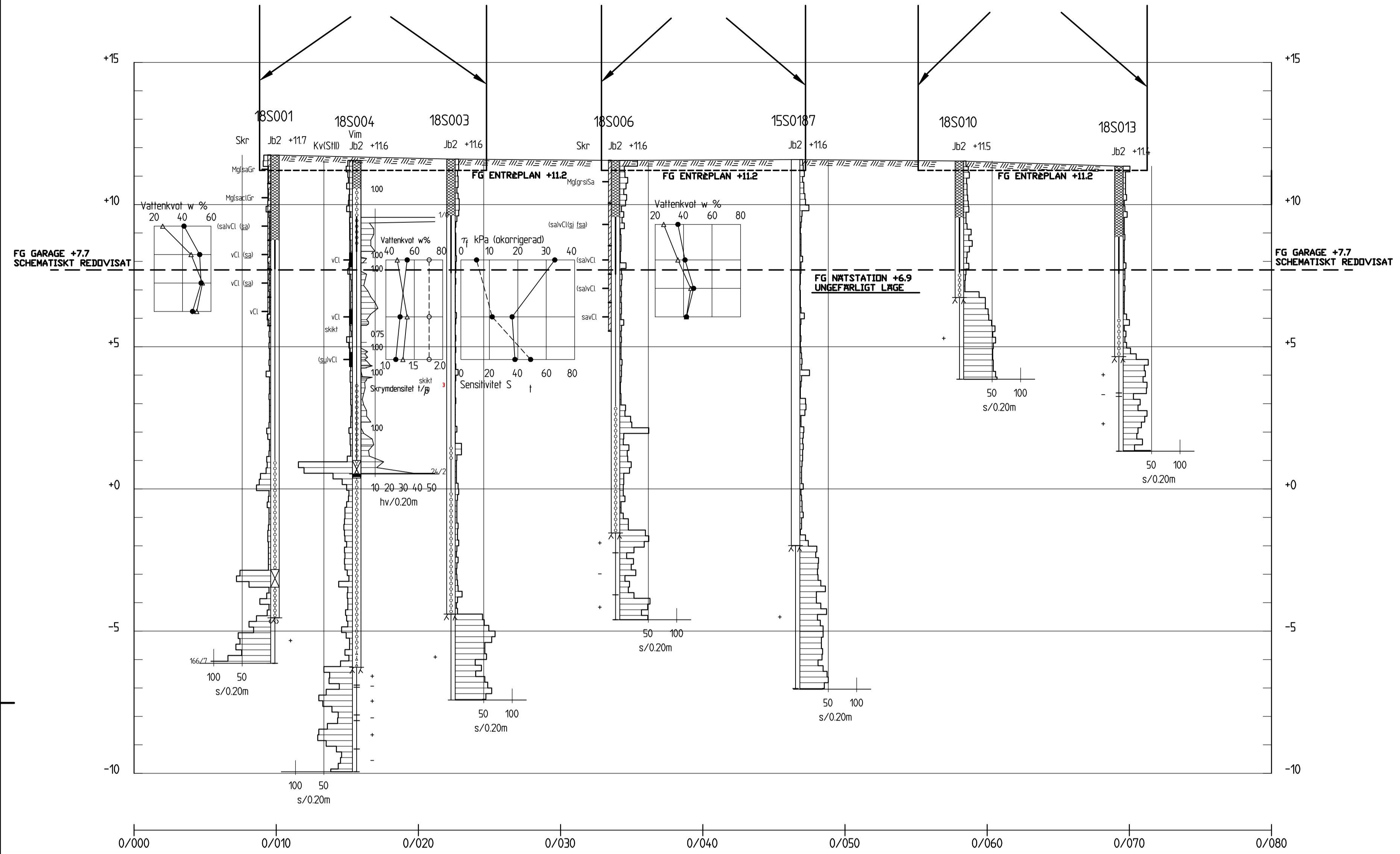
PROFIL C H 1:100 L 1:200
