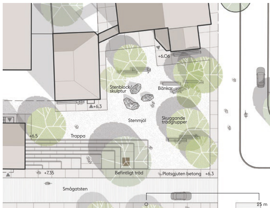
Situationsplan – ett parktorg med ett golv av stenmjöl och möblering under lövsugga (skala 1:500).
