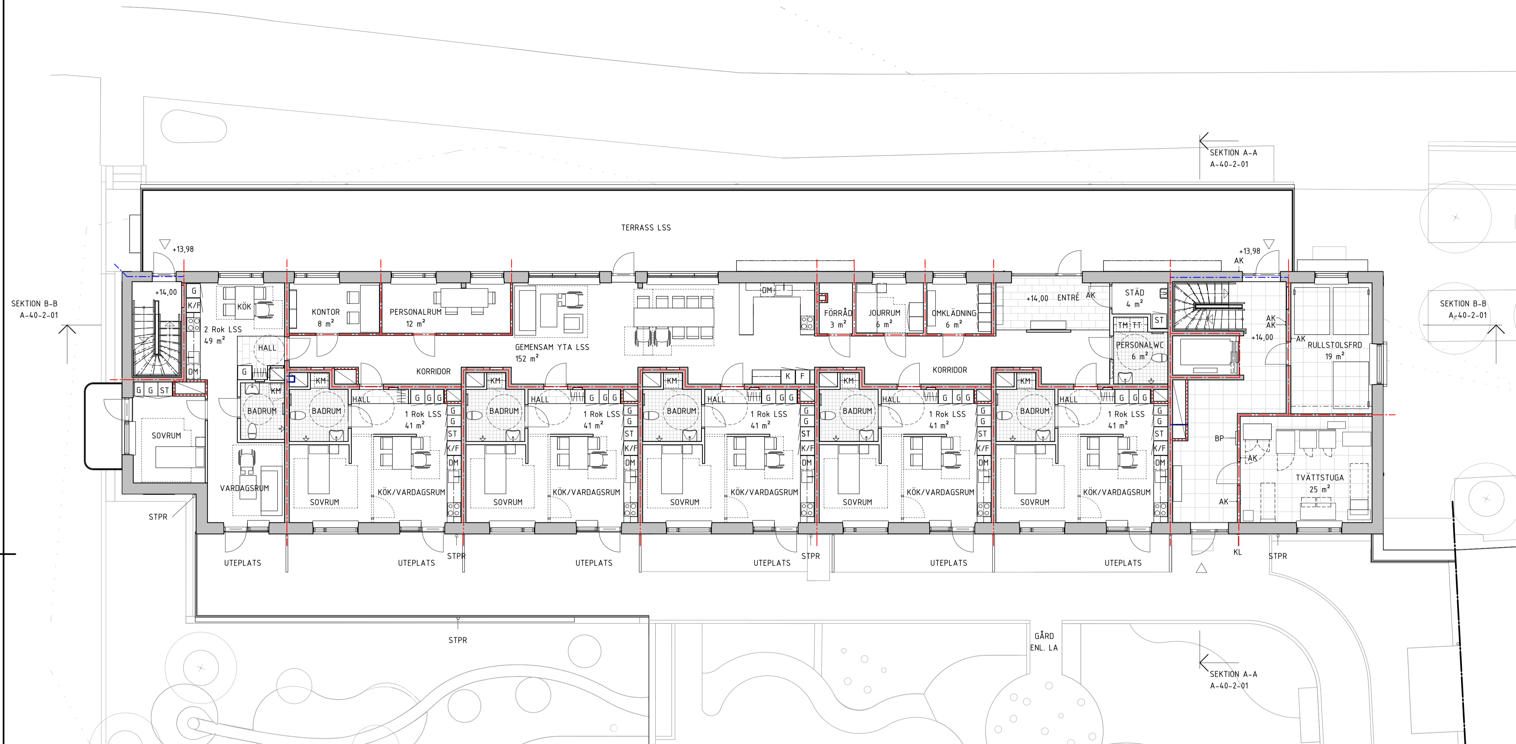
HUS 1 - PLAN 10.
