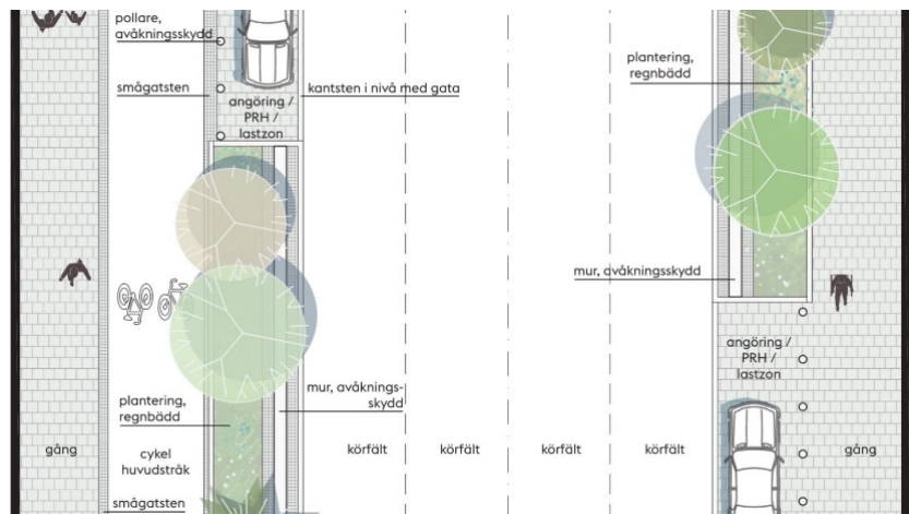
Planutsnitt Hammarbyvägen.
