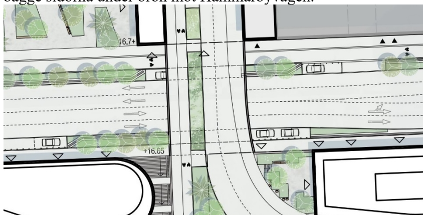
Den föreslagna bron över Hammarbyvägen (Illustration: Karavan landskapsarkitekter)
