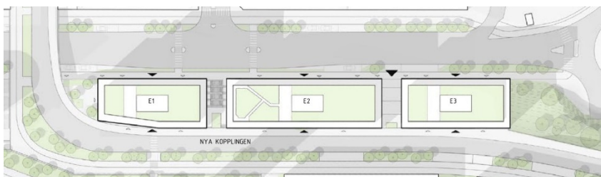
Situations- och takplan kvarter E. (Bild: Tham&Videgård)
