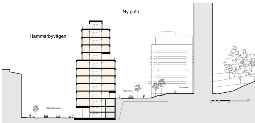
Sektion I-I, vy österut. (Bild: Tham&Videgård)
