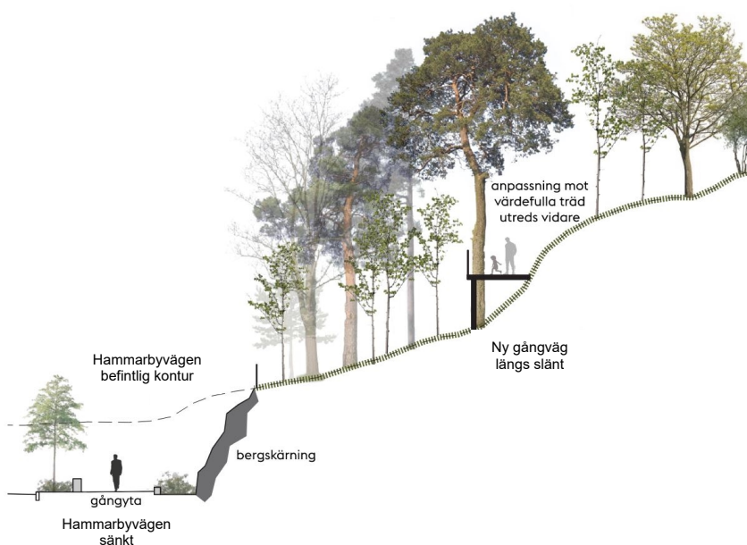
Principsektion som visar bergsskärning mot Hammarbyvägen och upphöjd gångväg i naturslätten mot söder.
