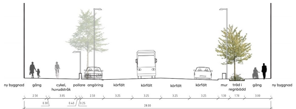
Principsektion Hammarbyvägen.
