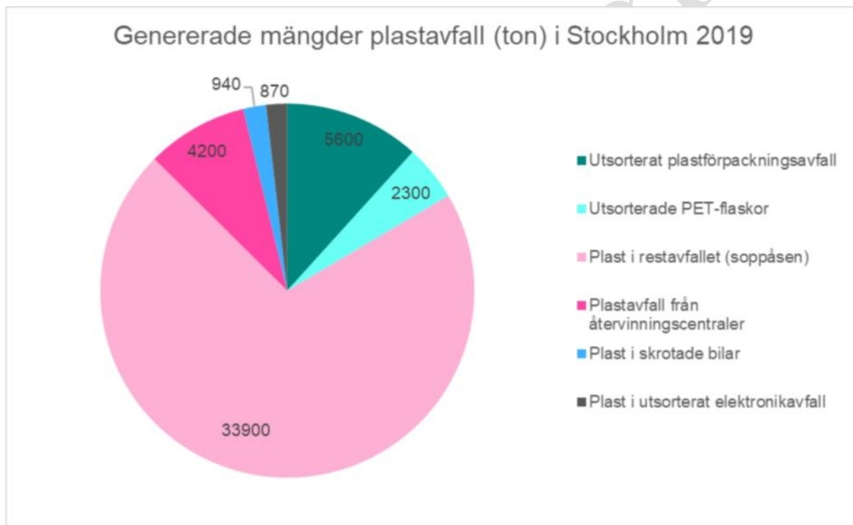
Figur 6. Genererade mängder plastavfall (ton) i Stockholm 2019 fördelat i olika produktkategorier. Denna figur kommer ersättas av en ny tillgänglighetsanpassad variant.
