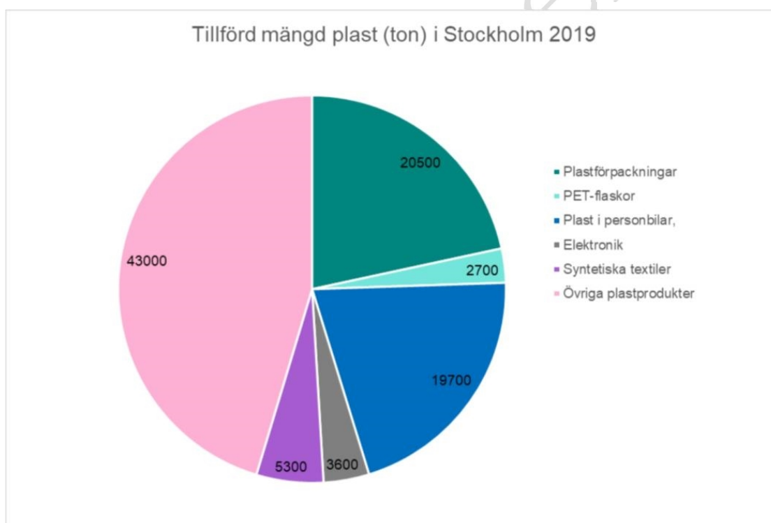
Figur 5. Invånarnas tillförda mängd plast (ton) under 2019 fördelat i olika produktkategorier. Denna figur kommer ersättas av en ny tillgänglighetsanpassad variant.
