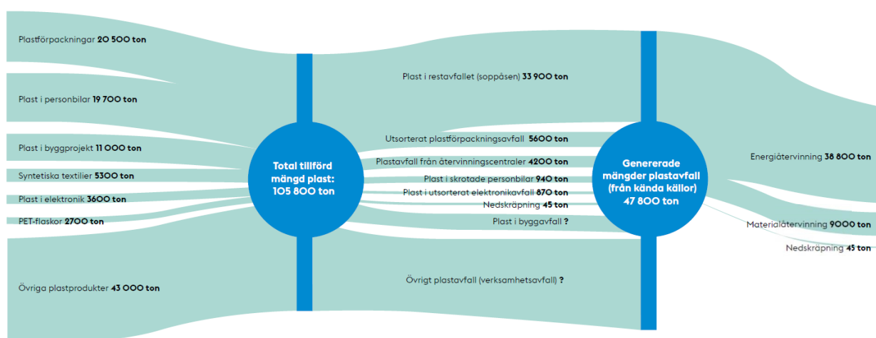
Figur 2. Under 2019 tillfördes Stockholm cirka 105 800 ton plast i form av olika varor, produkter och förpackningar. Drygt 11 000 ton plast uppskattats ha byggts in i byggprojekt. Uppskattningsvis genererades minst 47 800 ton plastavfall från olika varor, produkter och förpackningar, varav cirka 19 procent uppskattas ha gått till materialåtervinning och cirka 81 procent till avfallsförbränning. 45 ton plast har också uppskattats läcka ut som nedskräpning.
