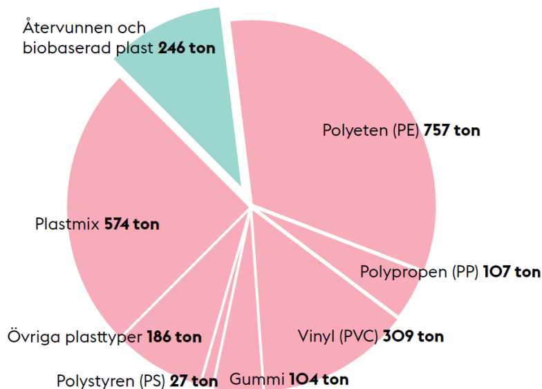
Figur 3. Uppskattade plastflöden från användning av utvalda förbrukningsartiklar (utifrån plasttyp) i Stockholms stad. Fossil plast dominerar bland de utvalda förbrukningsartiklarna, men en liten delmängd av artiklarna är tillverkade av återvunnen eller biobaserad plast.
