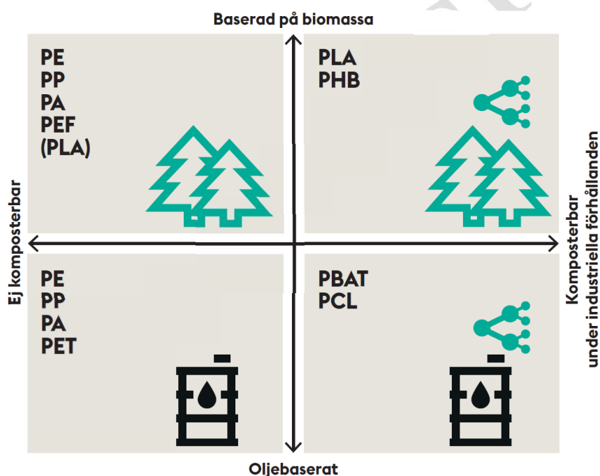
Figur 1. Figuren visar skillnaden mellan biobaserad och bionedbrytbar (komposterbar) plast. De traditionella plastsorterna PE (polyeten), PP (polypropen) och PA (polyamid) kan tillverkas både av biomassa och fossil olja. Andra plastsorter som PLA (polylaktid) och PHB (polyhydroxybuturat) tillverkas av biomassa och är bionedbrytbara (PLA kan dock göras mer eller mindre stabil). Det går också att tillverka bionedbrytbar plast av fossil olja exempelvis sorterna PBAT (polybutylenadipatereftalat) och PCL (polycaprolakton).
