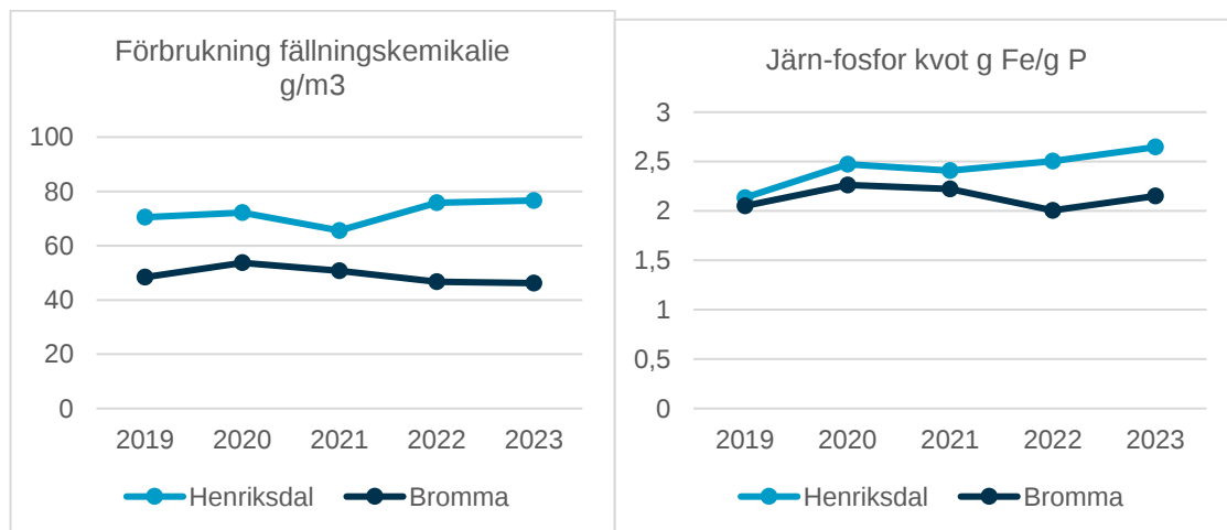
Figur 17. Förbrukningen av fällningskemikalie (g/m 3 ) i reningsverken under åren 2019-2023 samt kvoten tillsatt järn per inkommande fosformängd (g Fe/g P) under åren 2019-2023.
