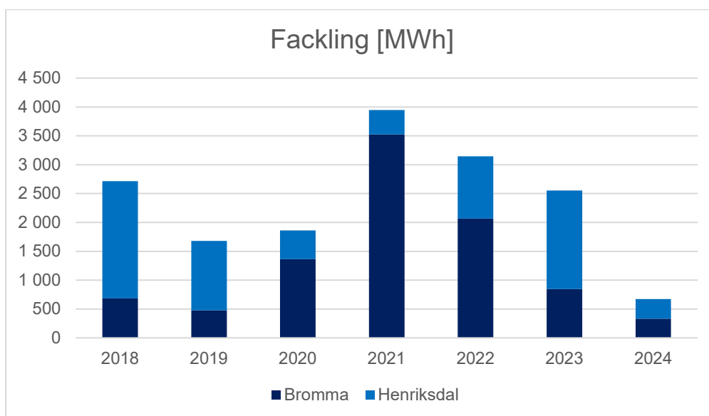
Figur 13 – Energinnehåll i facklad gas uppdelat per år mellan 2018-2024.
