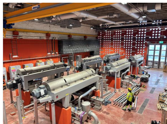
Figur 1. Slambyggnaden 2026–03. Stora centrifughallen.
