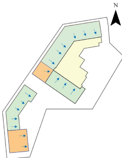
Avrinningspilar som visar avrinningen av dagvatten från taken. Grönt= vegetationsbeklätt tak, Orange= vanligt tak, ljusgult=markbeläggning, innergård (Funkia)
