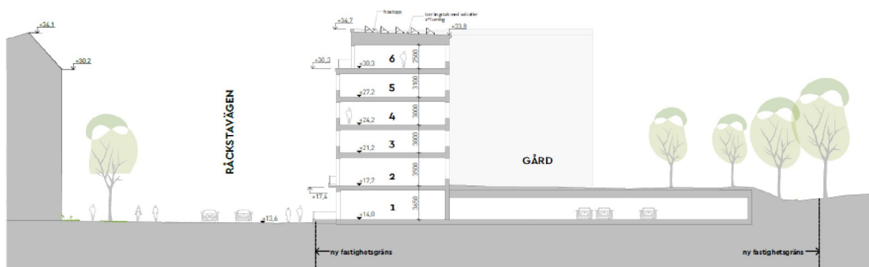
Sektion genom den norra byggnaden (Brunnberg & Forshed)
