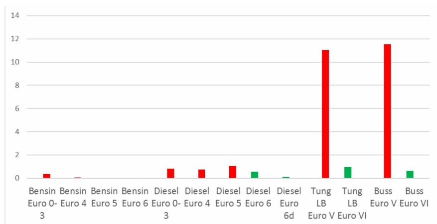
Figur 10: NO x g/km emissioner per fordon på Hornsgatans vägtyp. Diagrammet visar verkliga genomsnittliga utsläpp (enligt Hbefa 3.3, år 2017) inte normvärden. För jämförelsens skull är även personbilens utsläppen från föregående diagram medtagna.
